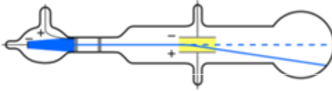
Crooken katodisädeputki, jota Thomson käytti elektronin massa/varaus suhteen määrittämiseen.
