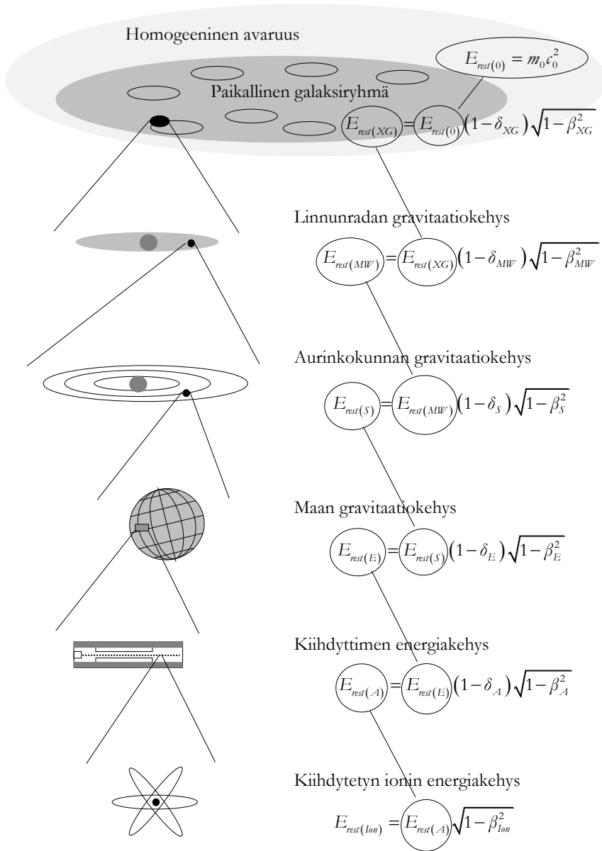
Kuva 3-7. Sisäkkäisten energiakeräysten järjestelmä. Jokainen energiakeräys sitoo osan objektin lepoenergiasta. Kiihdytetyn ionin energiatilaan ei liity gravitaatiotilan muutosta kiihdyttimessä, joten lepoenergiaa alentaa vain nopeustekijä. Kiihdyttimellä on sekä liike- että gravitaatiotila maapallon energiakeräyksessä, maapallolla auringon energiakeräyksessä, aurinkokunnalla Linnunradan energiakeräyksessä, Linnunradalla paikallisen galaksiryhmän energiakeräyksessä ja paikallisen galaksiryhmän energiakeräyksellä homogeenisessa avaruudessa.
