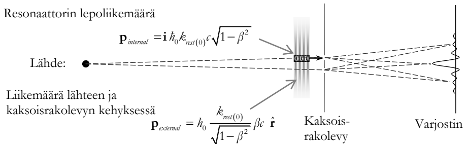
Kuva 3-9. Resonaattorina kuvattu objekti kaksoisrakokeksessä. Objektin rinnalla liikemäärää kuljettava massa-aalto läpäisee kummankin raon riippumatta siitä, kummasta raosta itse objekti kulkee. Varjostimella havaitaan liikemääräaallon synnyttämä interferenssikuvio.
