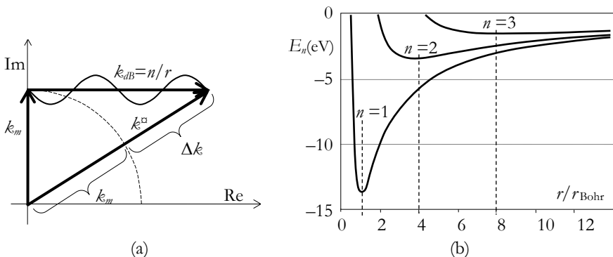
Kuva 3-10. Vetyatomien elektronin perustilat massa-aallon resonanssiehdosta ratkaistuna. (a) kompleksisen massa-aallon reaalikomponentin k_{dB}=n/r resonanssiehto. (b) Yhtälön (3.30) mukaiset kokonaisenergiat, kun n = 1, 2, 3 . Elektroni hakeutuu kullakin n:n arvolla yhtälön (3.31) mukaiseen energiatilan minimienergiaan, joka vastaa tarkalleen kvanttimekaniikan antamia energioita.
