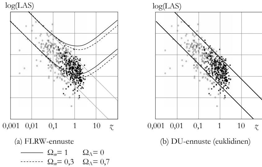
Kuva 3-17. Havaintoja galaksien (avoimet ympyrät) ja kvasaarien (mustat ympyrät) kulmakooosta (LAS) punasiirtyäalueella 0.001 < z < 3 111 . (a) FLRW-kosmologian ennusteet kaksille tiheysparametrien arvoilla. (b) DU-avaruuden euklidinen ennuste (3.22) vastaa hyvin havaintoja.
