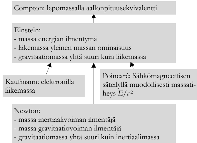
Kuva 2-3. Vaiheita massan määrittelyssä. Massan määrittely on Newtonin liikeyhtälöiden muotoilusta lähtien määrittynyt massan havaittujen ominaisuuksien perusteella. Tärkeimmät näistä ovat olleet inertiaaliominaisuus ja gravitaatio-ominaisuus. Lepomassan käsite johti tulkintaan massasta energian ilmenemismuotona.
