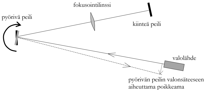
Kuva 1-22. Léon Foucault'n ja Hippolyte Fizeaun laitteisto valon nopeuden mittaamiseen 1850. Albert Michelson käytti samaan periaatteeseen perustuvaa laitteistoa vuonna 1883, jolloin hän sai valon nopeudeksi 299,864 \pm 51 km/s.
