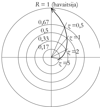
Kuva 3-16. Avaruuden 4-säteen R pituus ja kohteen sijainti punasiirtymillä z = 0 \dots 5 . Sijainti R = 1 on havaitsijan sijainti. Spiraalin muotoinen nuoli kuvaa valon etenemistä avaruuden laajetessa. Kuvassa valon, joka on lähtenyt liikkeelle R_4 -säteen ollessa 0,17, punasiirtymä on z = 5 valon edettyä matkan D = (1-0,17)R_4 laajenevassa avaruudessa.
