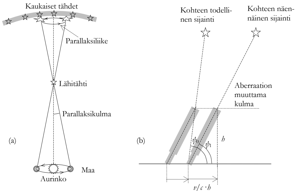
Kuva 1-11. (a) Jos maan oletetaan kiertävän aurinkoa, pitäisi lähellä olevien tähtien näennäisen sijainnin kaukana oleviin tähtiin nähden muuttua vuoden aikana parallaksin vuoksi. Tyko Brahen aikaisilla havaintovälineillä parallaksin havaitseminen ei ollut mahdollista. (b) Kohteen kulmamittauksessa mitaajan nopeus synnyttää aberraation seurauksena havaintokulmaan näennäisen poikkeaman kohteen todelliseen sijaintikulmaan. Havaintoon käytetyn kaukoputken edetessä nopeudella v vertailutasossa kohti, on kaukoputkea kallistettava kulmaan \psi_1 , jotta kaukoputken yläpäähän osuva valo saavuttaa havaitsijan putken alapäässä. Aberraation selitti englantilainen astronomi James Bradley 1700-luvulla.
