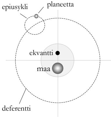
Kuva 1-4. Episyklisysteemin rakenne. Planeetan radan määrää kiertoliike episyklillä, joka puolestaan kiertää deferenttiä myöten tasaisella kulmanopeudella ekvanttiin nähden. Deferentin keskipiste ei ole maa, vaan maan ja ekvantin puolivälissä oleva piste.
