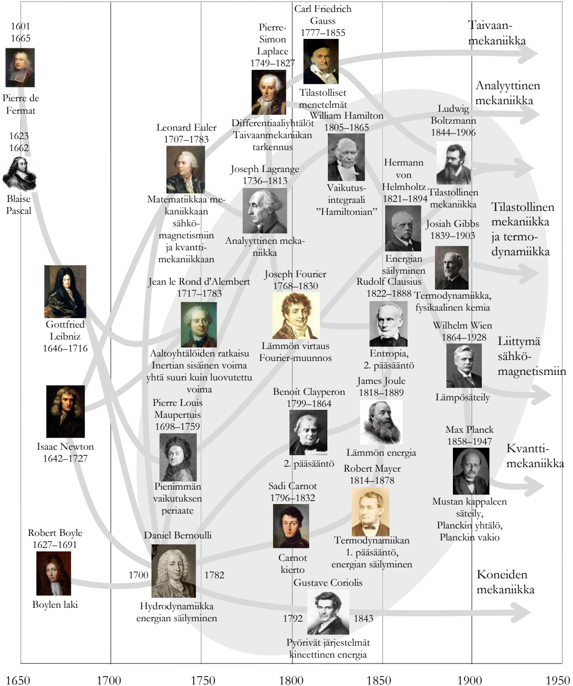
Kuva 1-16. Newtonin jälkeen tapahtunut mekaniikan kehitys ja kehityspolkujen jakautuminen mekaniikan eri osaluoksiin. Kehityksessä yhdistyi 1700-luvun matematiikan voimakas kehitys ja toisaalta 1800-luvulle painottunut vahvasti empiirinen tutkimus. 1800-luvun empirismiä täydensi sähkömagnetismi, joka ennen kaikkea energiäkäsitteen kautta kytkeytyi mekaniikan tuloksiin. Harmaa taustaellipsi kuvassa kuvaa aluetta, jossa painottuu energiäkäsitteen selkiytyminen ja energian säilyminen perustavaa laatua olevana luonnonlakina.
