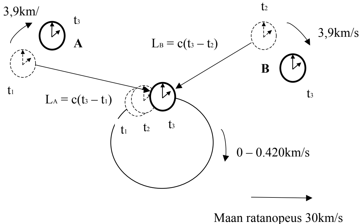
Kuva 4. GPS-järjestelmän periaate
