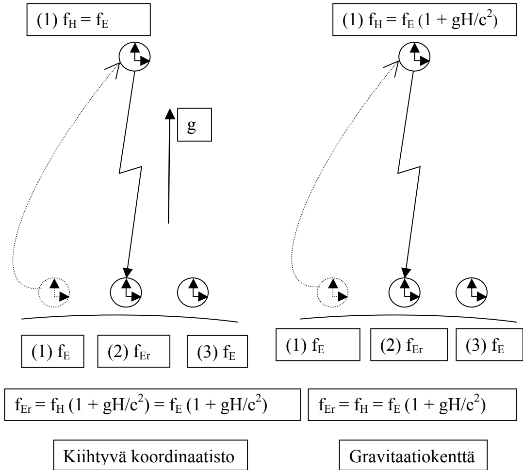
Kuva 1. Ekvivalenssiperiaate.
