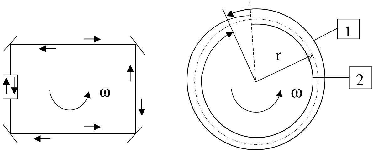
Kuva 3. Sagnac-koe.
